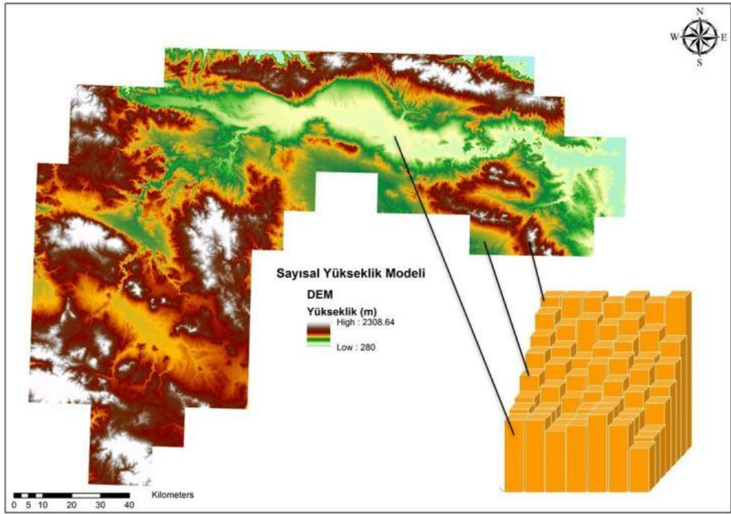
Şekil 2.7. DEM'in hücresel şekli ile ifadesi.
