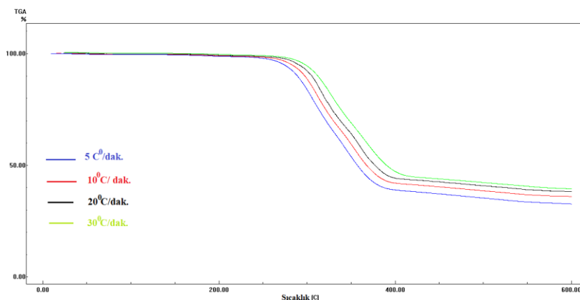
Şekil. Poli(ε-CL-co-BMA)'nın farklı sıcaklıklarda TGA Spektrumları
