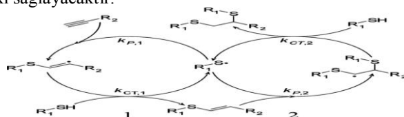
Şekil 1: Tiyol-in mekanizması
