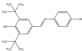
Şekil 2. Kullanılan organik maddenin kimyasal yapısı
