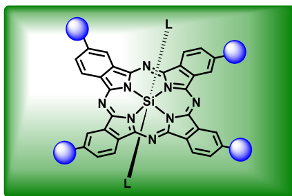
Şekil 1: Hedef Süstitüe Silisyum(IV) Ftalosiyanimin Gösterimi
