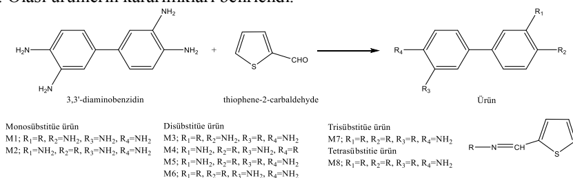
Şekil 1. Sentezi tasarlanan olası ürünler.
