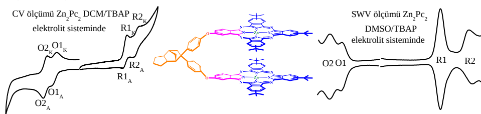
Şekil 1. Dinükleer Çinko Ftalosiyenin Bileşiğinin farklı çözücü ortamlarında kaydedilen CV ve SWV ölçümleri.
