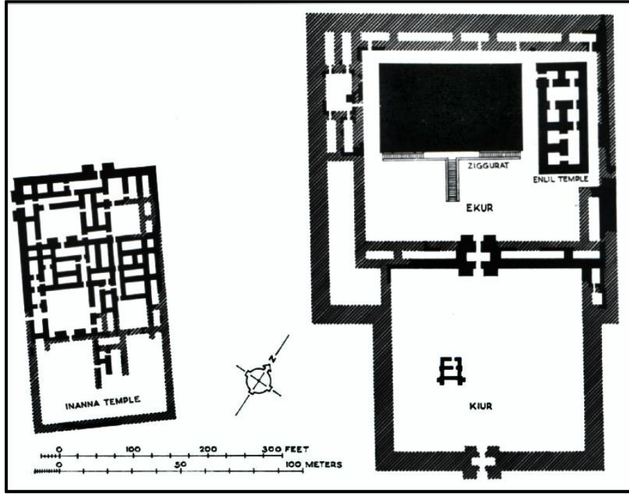
Resim 11: Nippur Kenti İnanna Tapınağı Planı Kaynak: Crawford, 1959: 74'den düzenlenmiştir.
