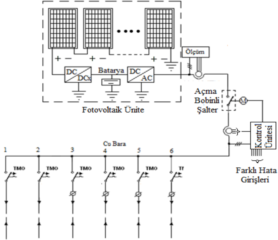
Şekil 5.6. Sistemin fotovoltaik bir üniteye uygulanması.
