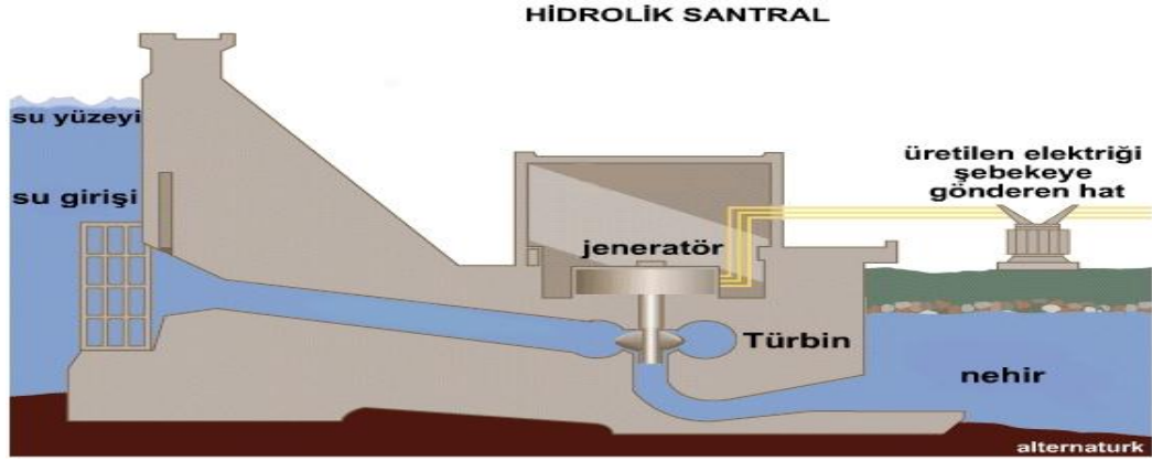
Şekil 2.4. Hidroelektrik santral.
