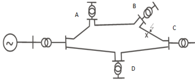
Şekil 2.14. Ring şebeke.
