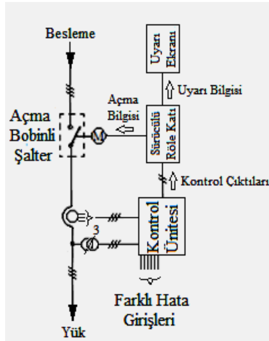
Şekil 5.3. Uygulama akış devresi.
