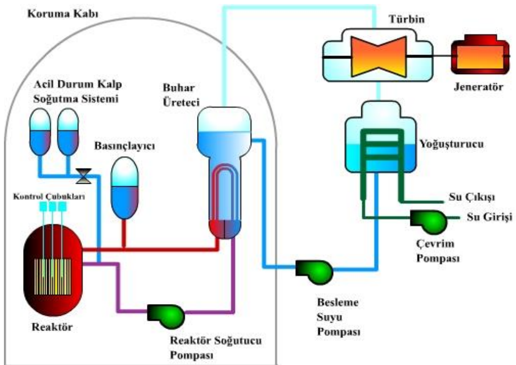
Şekil 2.8.PWR çalışma diyagramı
