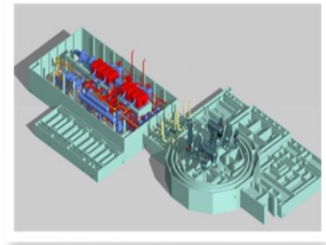
Şekil 2.14. VVER -1200 tasarımı nükleer reaktör simülasyonu
