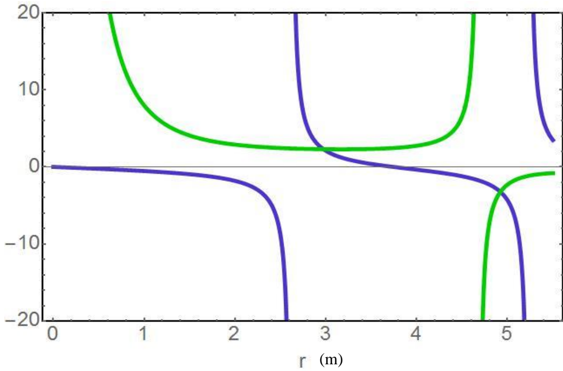
Şekil 3.10: \mu=1.2 ve \nu=1.2 için 7. denklemin sağ (yeşil eğri) ve sol taraflarının (mavi eğri) r 'nin fonksiyonu olarak grafiği
