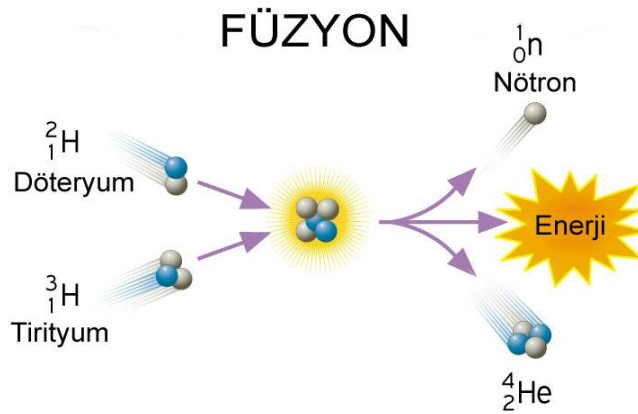
Şekil 2.2. Füzyon Reaksiyon
