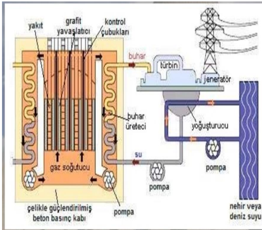
Şekil 2.10. Gaz soğutmalı reaktör blok diyagramı
