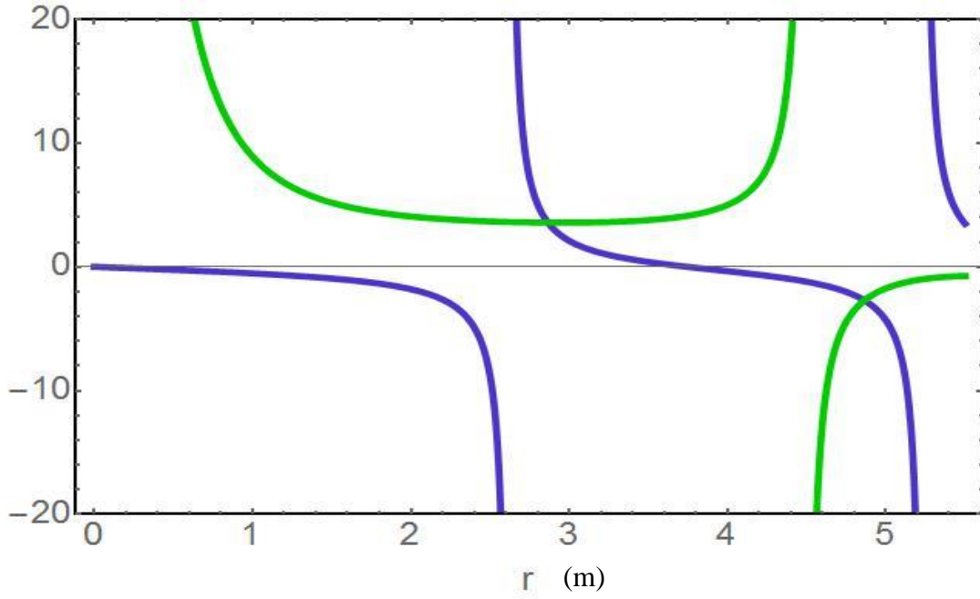
Şekil 3.9: \mu=1.2 ve \nu=1.8 için 7. denklemin sağ (yeşil eğri) ve sol taraflarının (mavi eğri) r 'nin fonksiyonu olarak grafiği.
