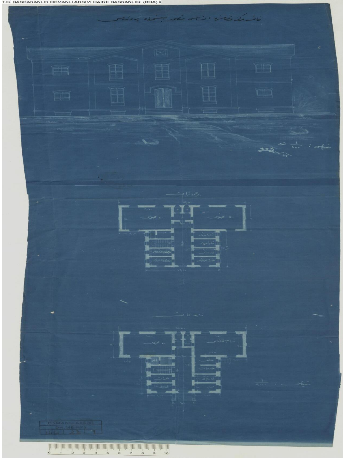
EK-II: Fatsa'da inşa edilecek hapishanenin keşif planı. BOA. DH. HPS.144.23.1
