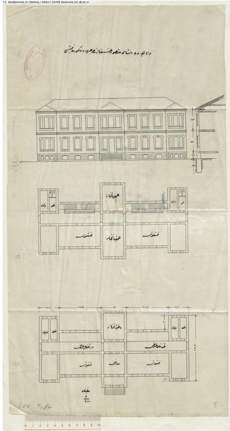
Germiyan Vakfi Tarafından Kütahya'da Yapımına Karar verilen Hastahänenin Planı
