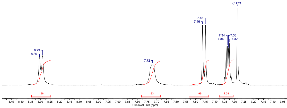
Bileşik A3 ^1\text{H-NMR} Spektrumu ( \text{CDCl}_3 , 500 MHz)
