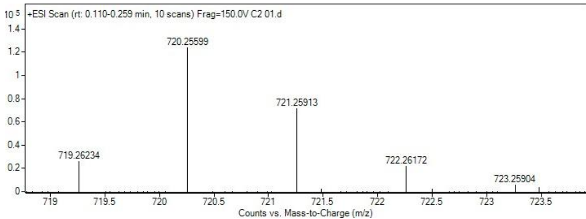
Bileşik C2 HRMS-TOF-ESI Spektrumu
