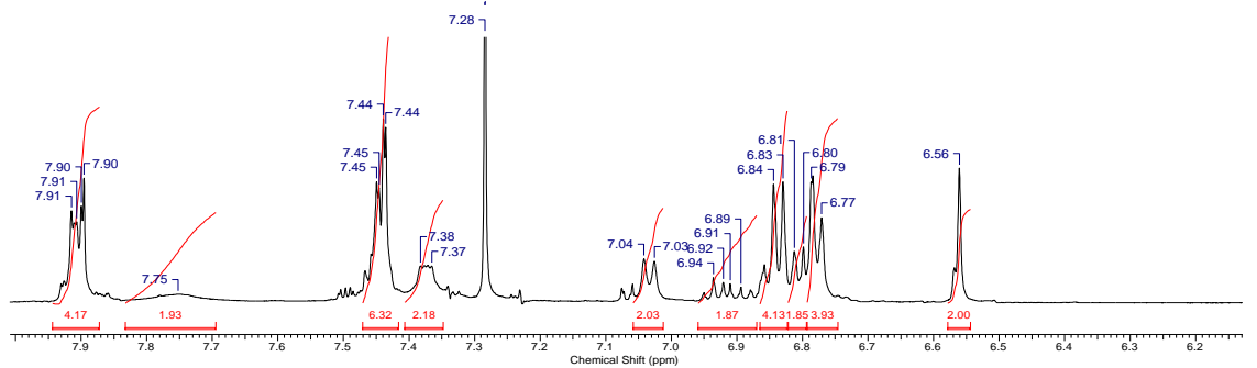
Bileşik B3 1 H-NMR Spektrumu (CDCl 3 , 500 MHz)
