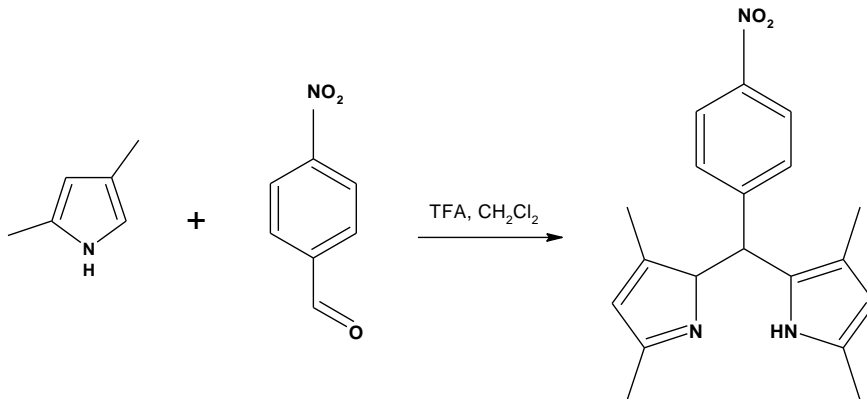
Şekil 2.4. Bordipirometen bileşiklerinin sentezinde sübtitüe pirol kullanımı, örnek reaksiyon
