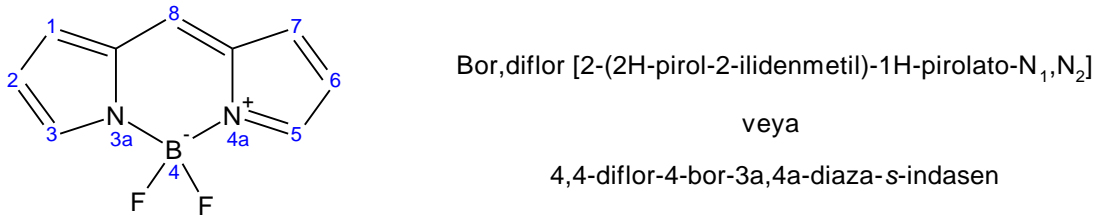
Şekil 2.2. BODIPY çekirdeğinin adlandırılması
