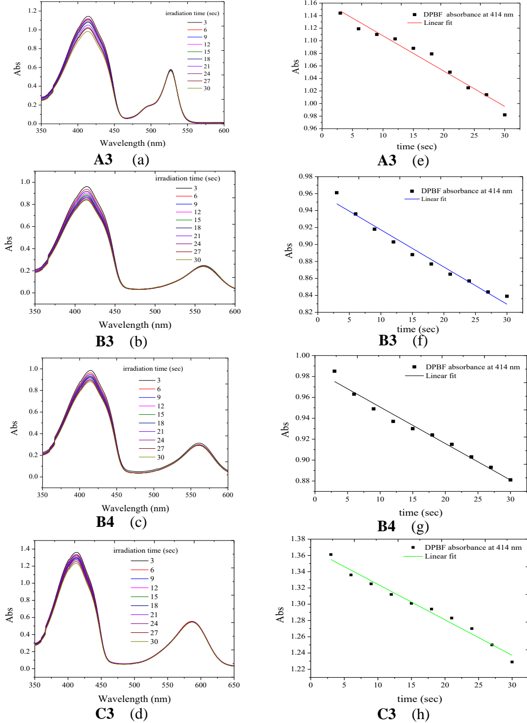
Şekil 5. 1. BODIPY-benzimidazol türevlerinin DPBF bileşiminin 414 nm absoransı üzerindeki etkileri
