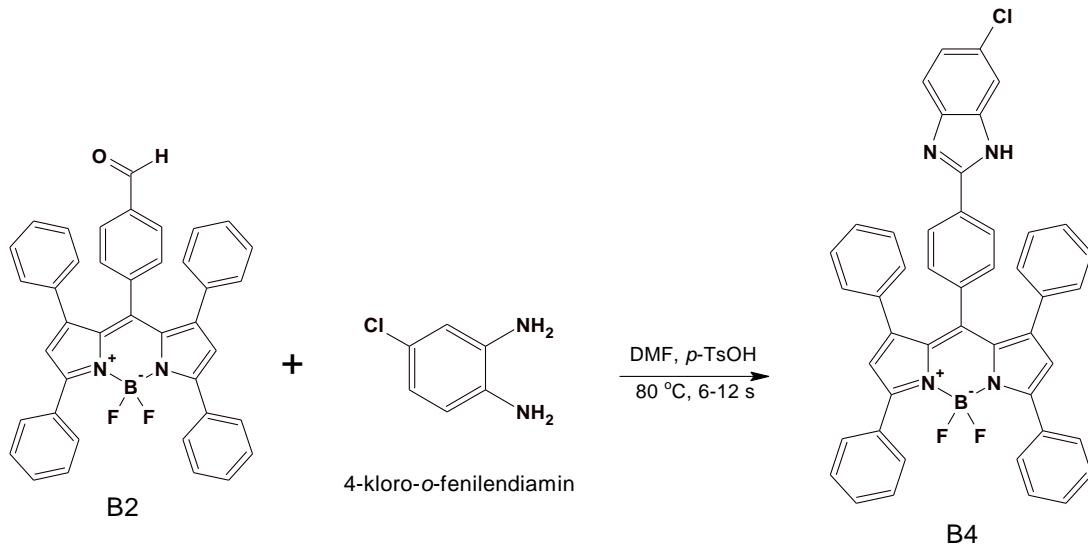
Şekil 4.9. B4 Bileşiğinin Sentez Yöntemi
