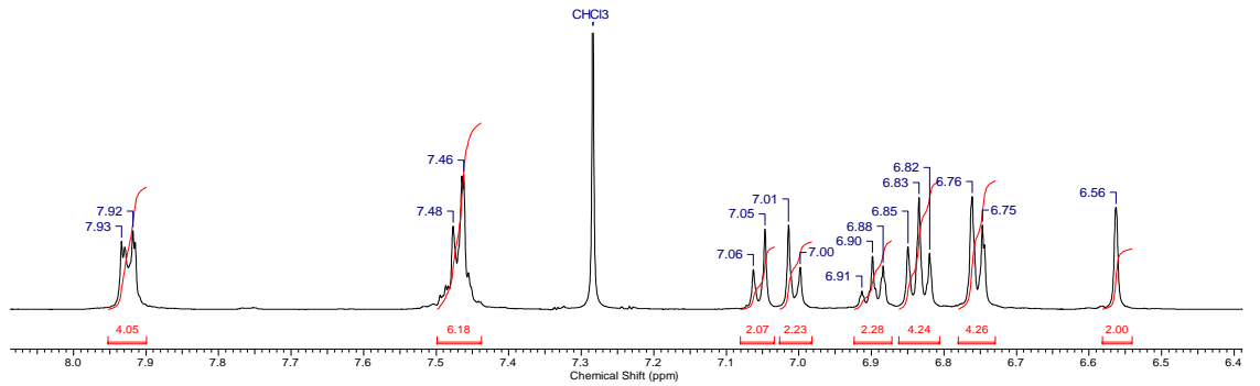
Bileşik B2 1 H-NMR Spektrumu (CDCl 3 , 500 MHz)
