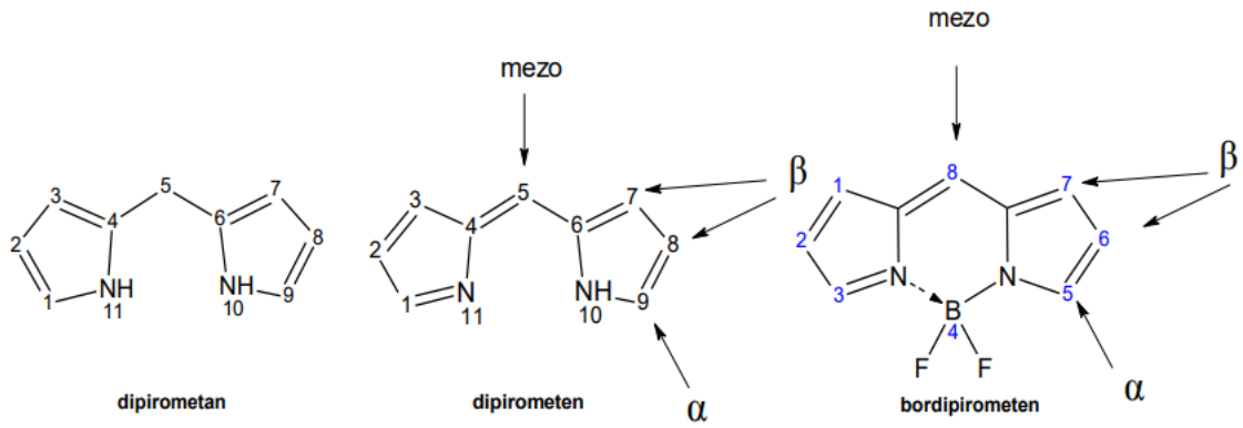
Şekil 2.1. Dipirometan, dipirometen, BODIPY bileşiğinin numaralandırması
