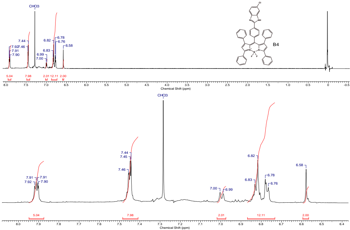
Bileşik B4 1 H-NMR Spektrumu (CDCl 3 , 500 MHz)
