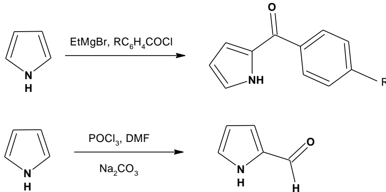
Şekil 2.7. Karbonilpirollerin sentezi
