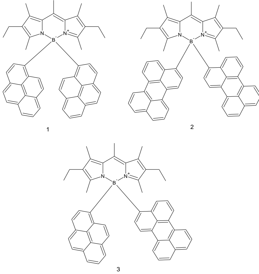
Şekil 2.15. Örnek BODIPY tabanlı enerji transfer kaseti
