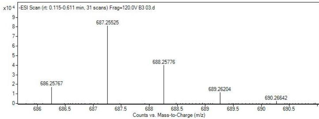
Bileşik B3 HRMS-TOF-ESI Spektrumu
