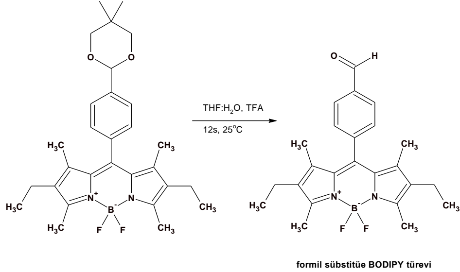
Şekil 3.3. Formil süstitüe BODIPY türevinin sentezi
