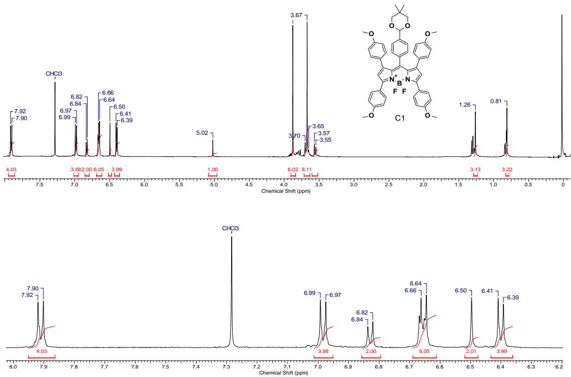
Bileşik C1 1 H-NMR Spektrumu (CDCl 3 , 500 MHz)
