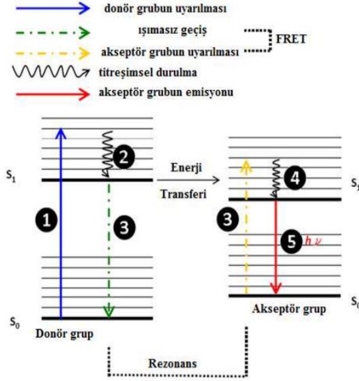
Şekil 2.12. Floresans rezonans enerji transferi (FRET)
