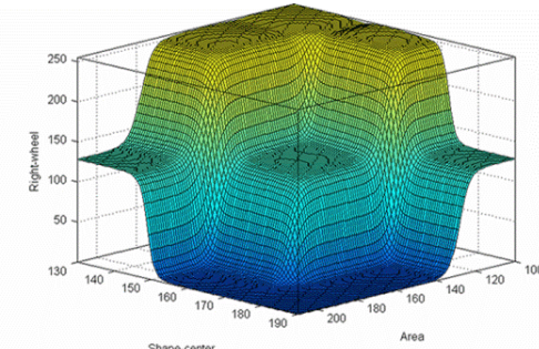
(b): Sağ teker kontrol yüzeyi.
