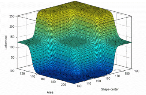
(a): Sol teker kontrol yüzeyi.
