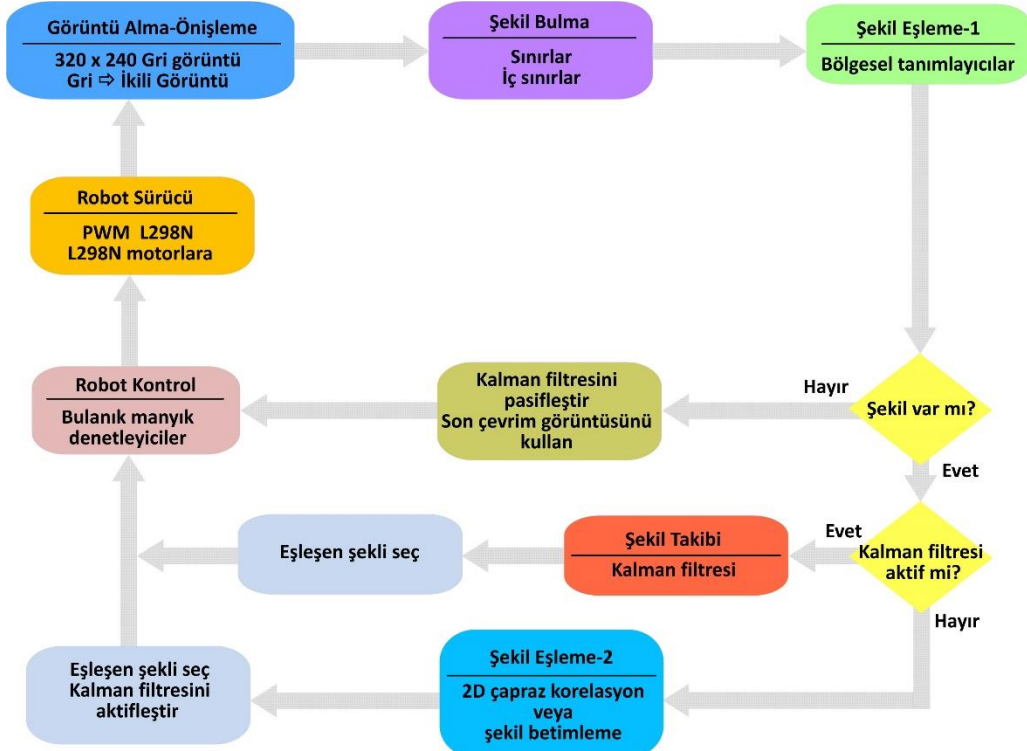
Şekil 5: BLMp'nun lider takip şeması.
