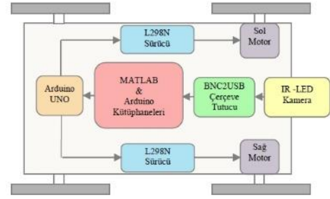
Şekil 3: BLMp'nun donanım yapısı.
