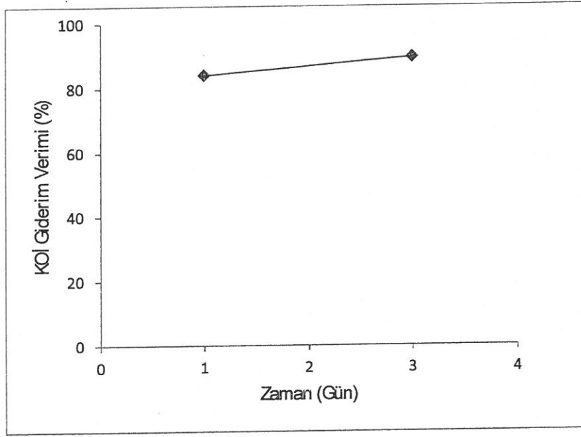
Şekil 4. KOİ giderim verimi
