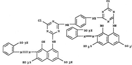
Şekil 1. Ostazin Black H-N açık kimyasal formülü
