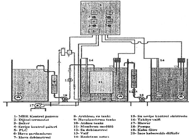
Şekil 2. MBR sisteminin şematik gösterimi
