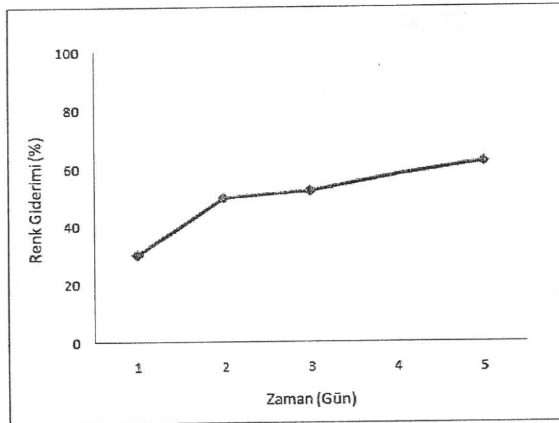
Şekil 3. Ostazin Black HN reaktif boya giderim verimi
