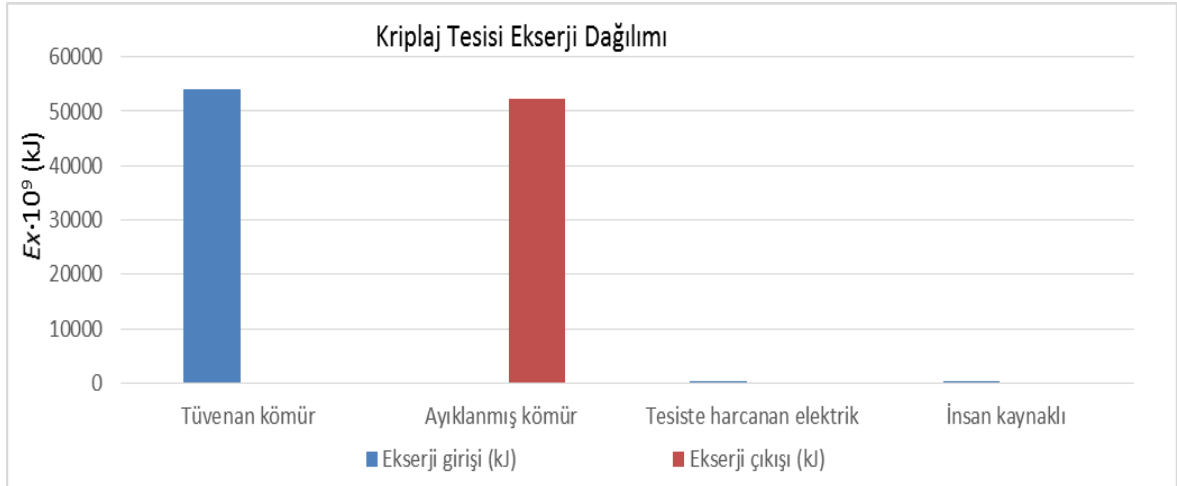
Şekil 7. Kriplaj tesisi enerji dağılımı. (Exergy distribution of coalbreaking.)
