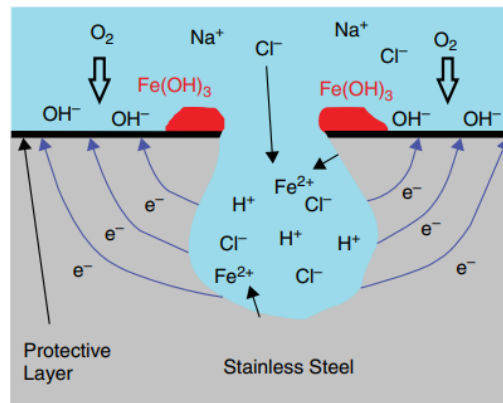
Şekil 2.5. Çukur korozyon oluşumu (Nazari, vd., 2018).
