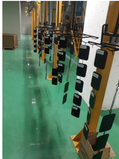
Şekil 4.8. Yüksek sıcaklık fırınında kürlenme süreci tamamlanan plakalara ait fotoğraf.
