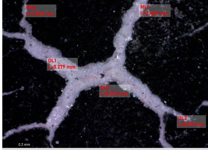
Şekil 6.14. Başarısız olarak değerlendirilen 1NA40 numunesine ait darbe testi görüntüsü.
