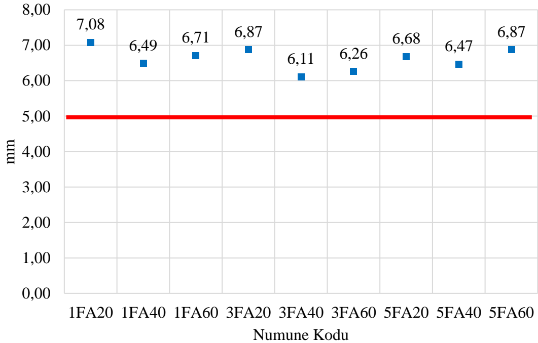
Şekil 5.9. Formik asit ile pasive edilen plakaların cupping direnci deęerleri.
