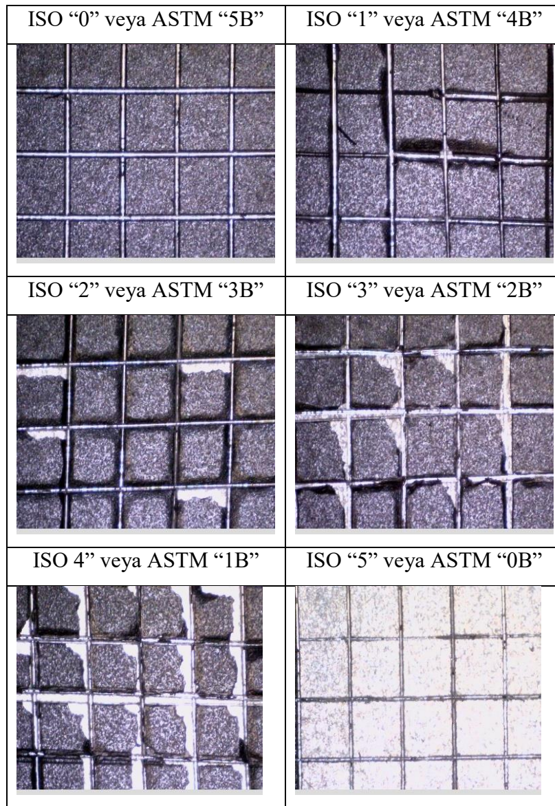
Şekil 6.1. ISO ve ASTM standartlarına göre cross-cut testi değerlendirmesine ait fotoğraf.
