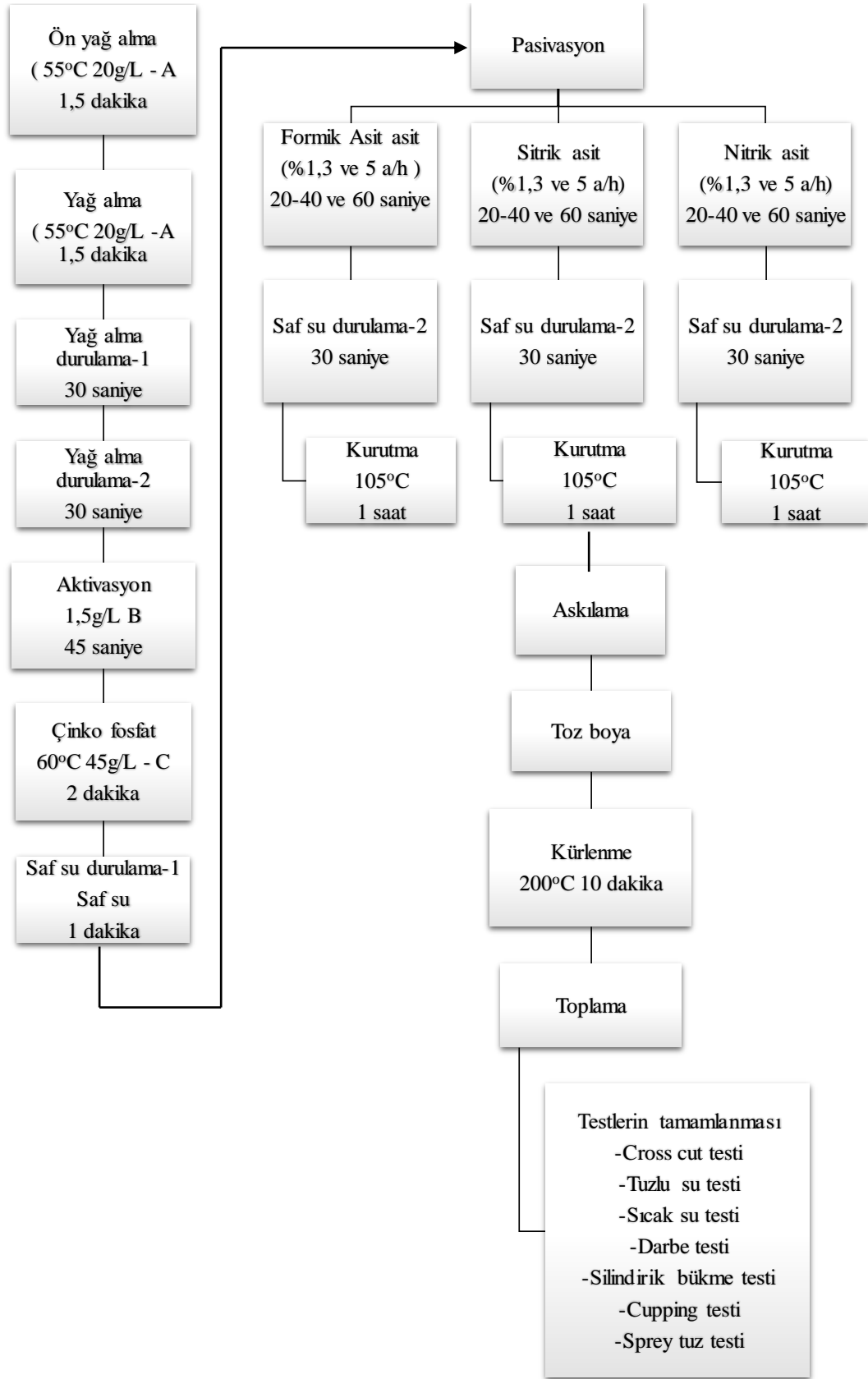
Şekil 4.1. Galvaniz sacların yüzey işlemleri süreci akış şeması.
