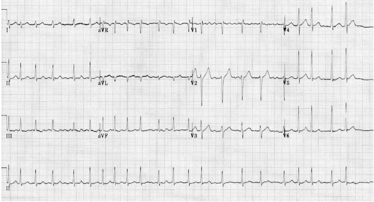
Şekil 2.30. Atriyal Fibrilasyon EKG Örneği
