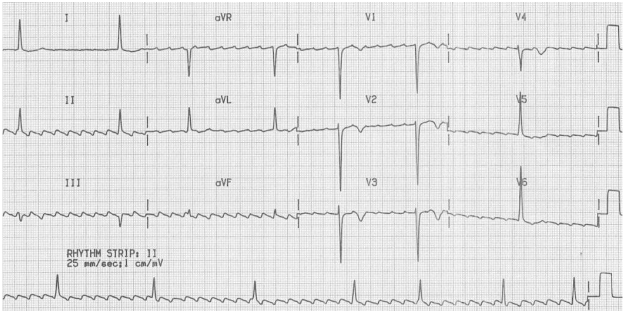
Şekil 2.28. Atriyal Flutter EKG Örneği
