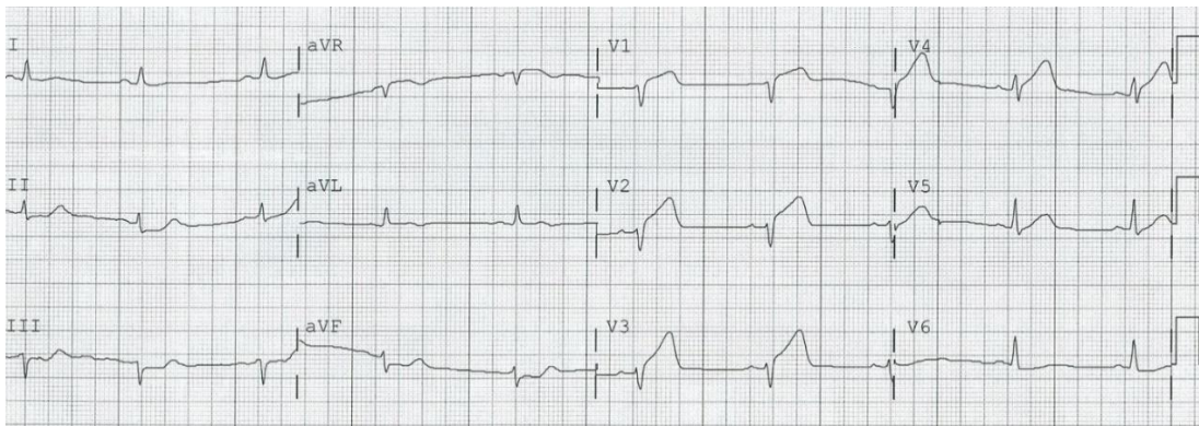
Şekil 2.18. Anterior STEMI EKG Örneği
