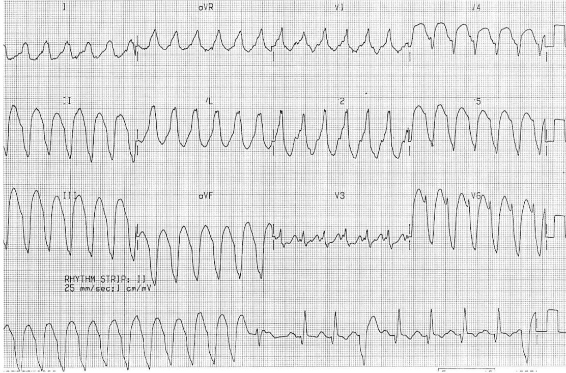
Şekil 4.14. Ventriküler Taşikardi EKG örneği
