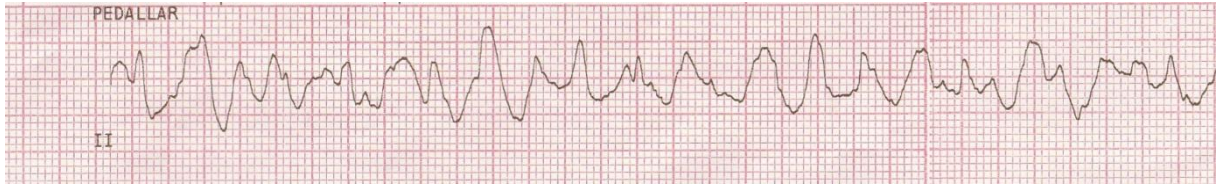
Şekil 2.24. Ventriküler Fibrilasyon EKG Örneği
