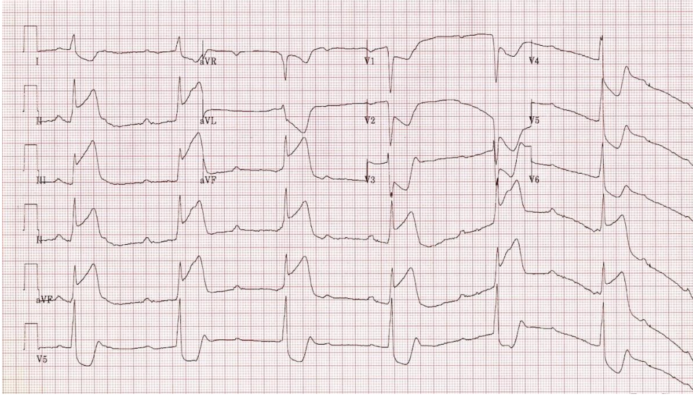
Şekil 2.13. 3. Derece AV Tam Blok
