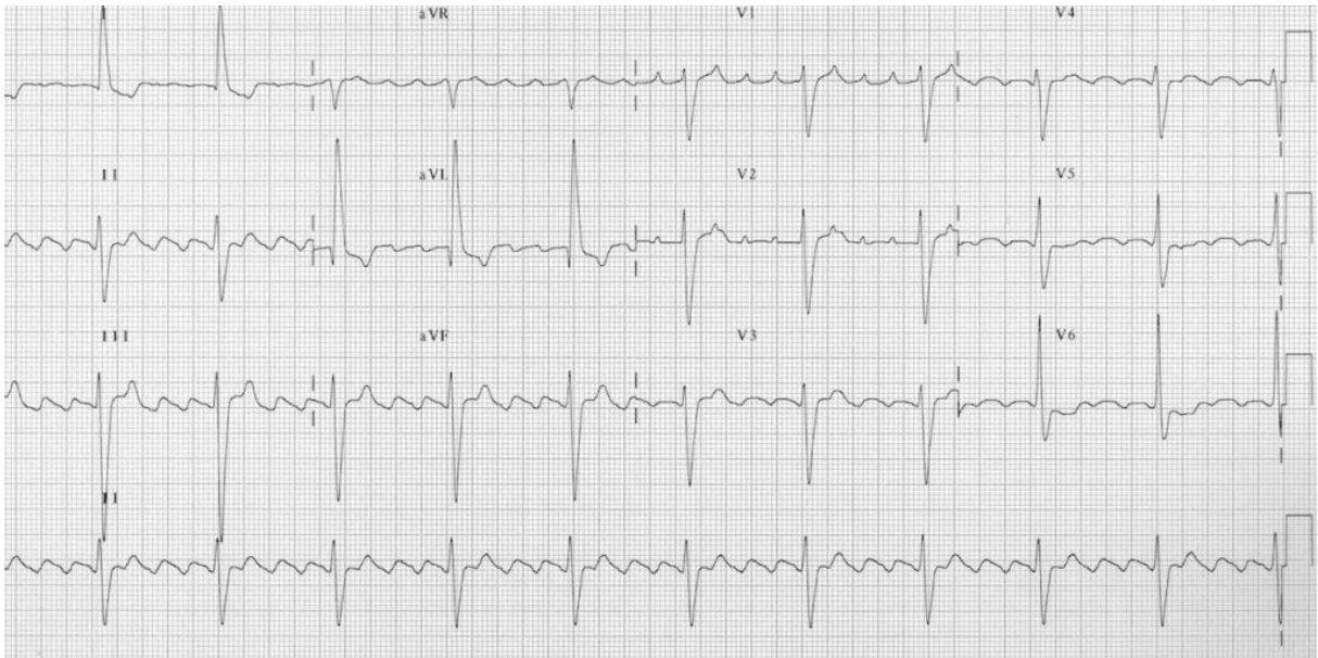
Şekil 4.8. Atriyal Flutter EKG örneđi
