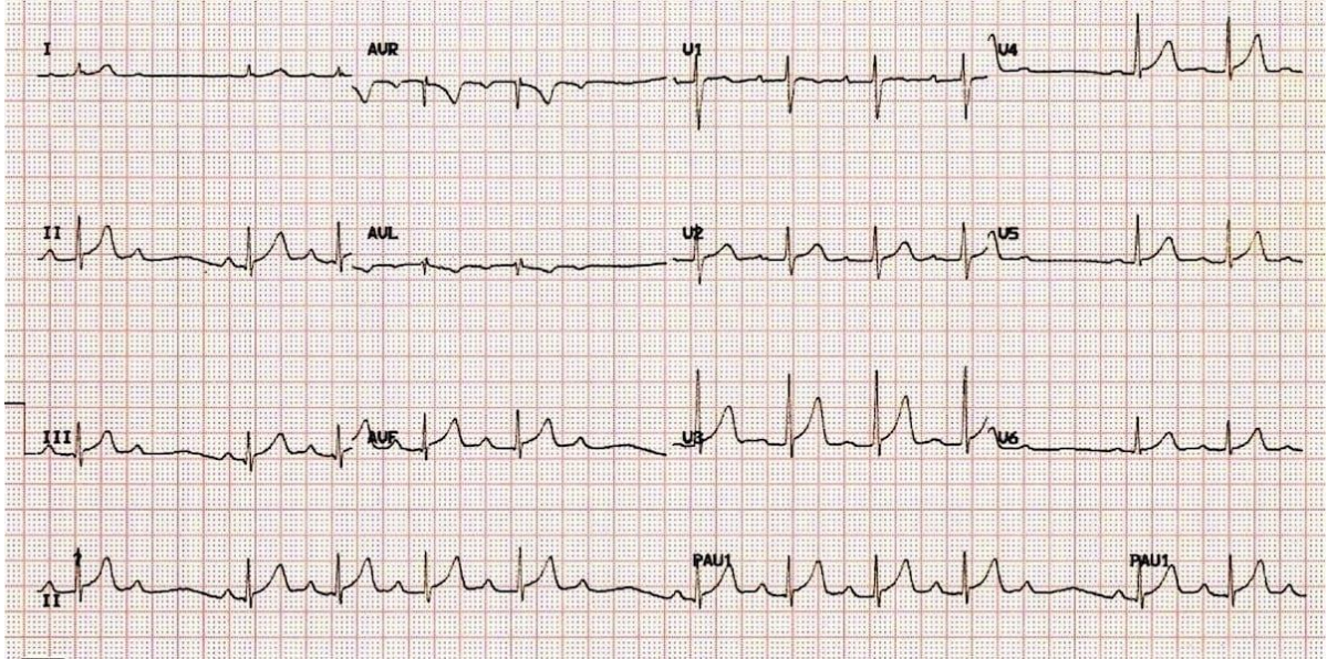
Şekil 2.11. 2. Derece AV Blok Mobitz Tip 1
