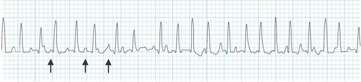
Şekil 2.29. Multifokal Atriyal Taşikardi EKG Örneği
