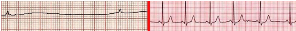
Şekil 2.22. Nabızsız Elektriksel Aktivite EKG Örneği
