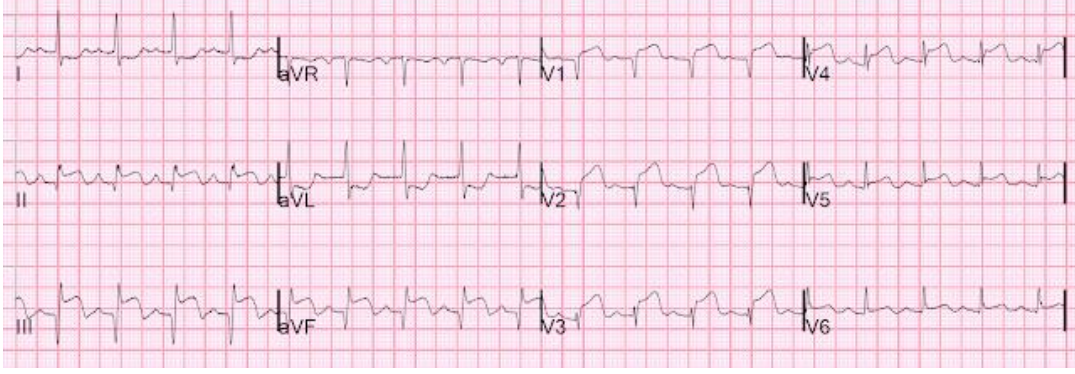
Şekil 2.16. Sağ Ventrikül Myokard İnfarktüsü
