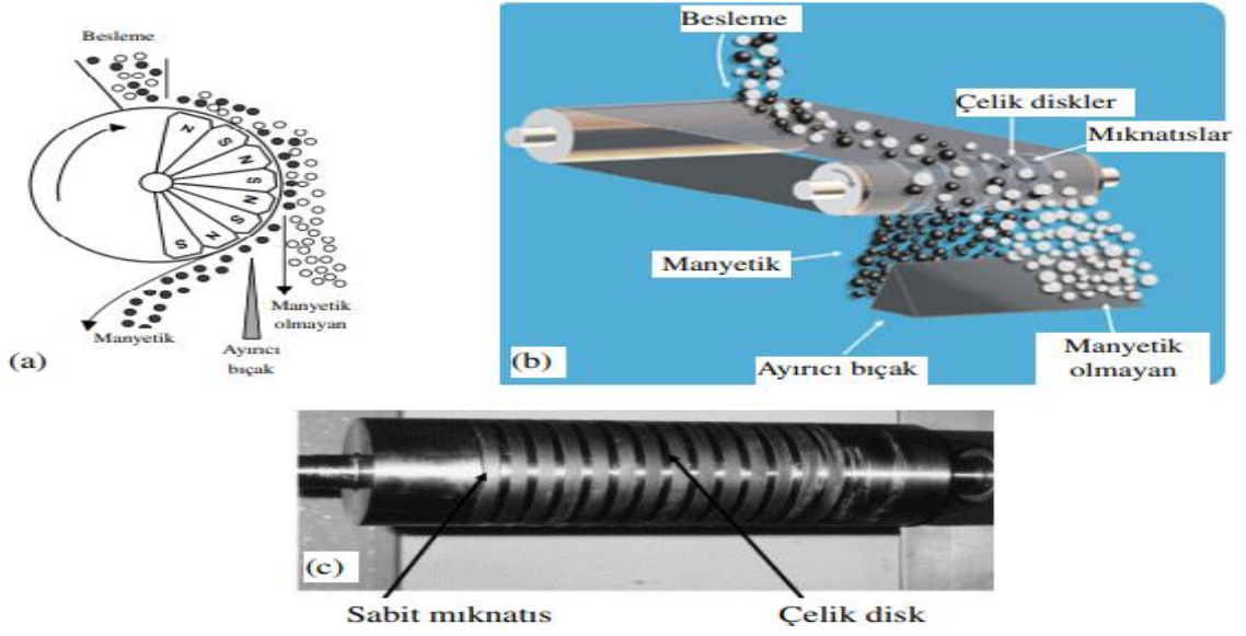
Şekil 3.17. Sabit Miknatslı Ambur Tipi Rulo Tipi Manyetik Ayırıcı (Rulo Tipi Ayırıcılarda Kullanılan Sabit Miknatslı Tambur)
