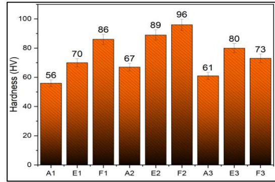
Şekil 6. Mikro Sertlik Sonuçları (HV) (Microhardness Results)
