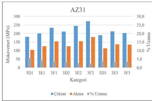
Şekil 7. Çekme Dayanımı, Akma Sınırı, % Uzama. (Tensile Strength, Yield Strength, %Elongation.)
