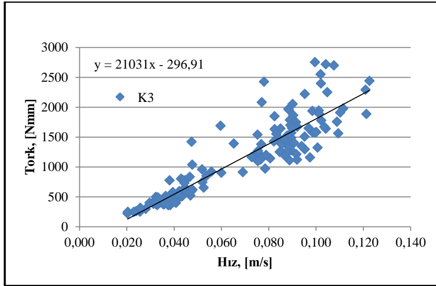
Şekil 4. 6. K3 reometre sonucu.
